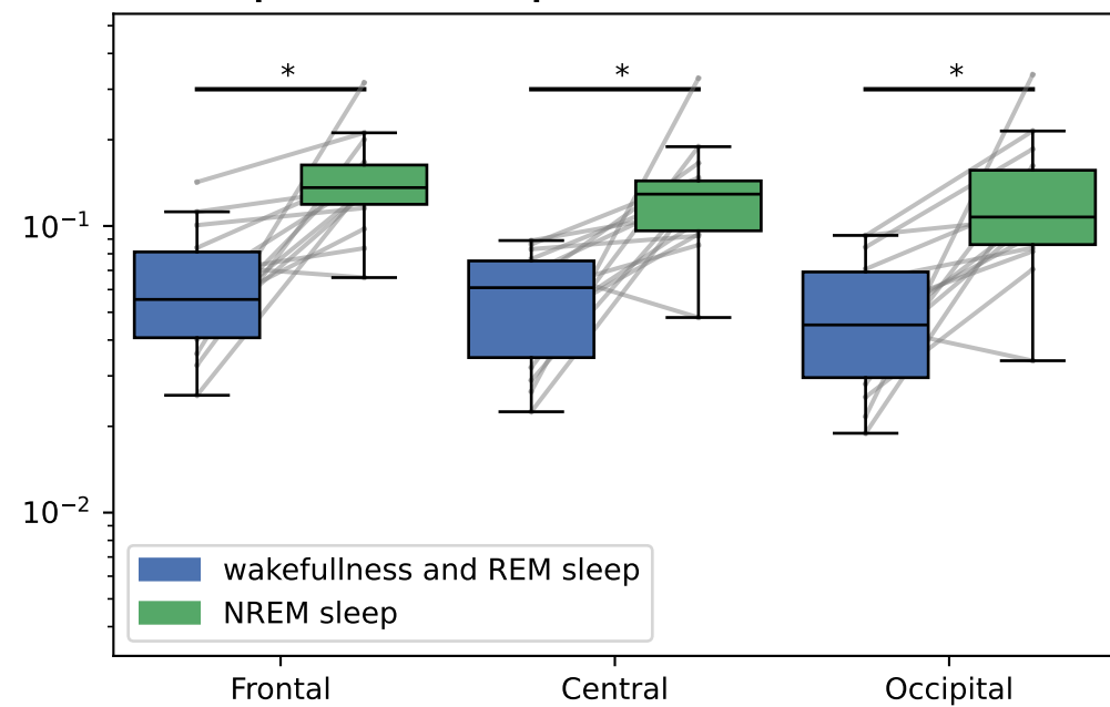
(D) Mean wPLI for Spindles
