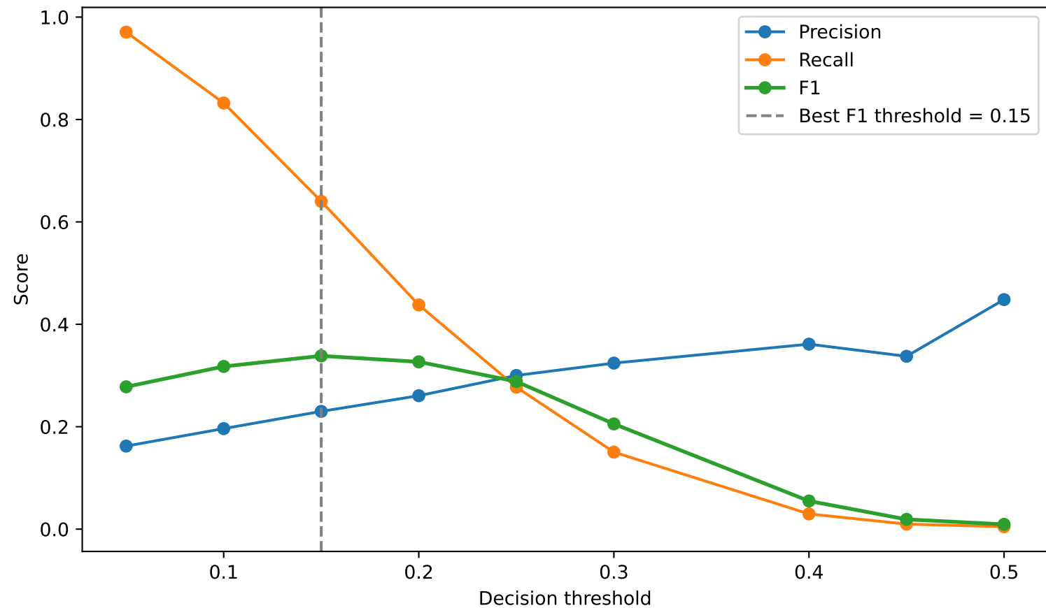
Precision / Recall / F1 vs. classification threshold
