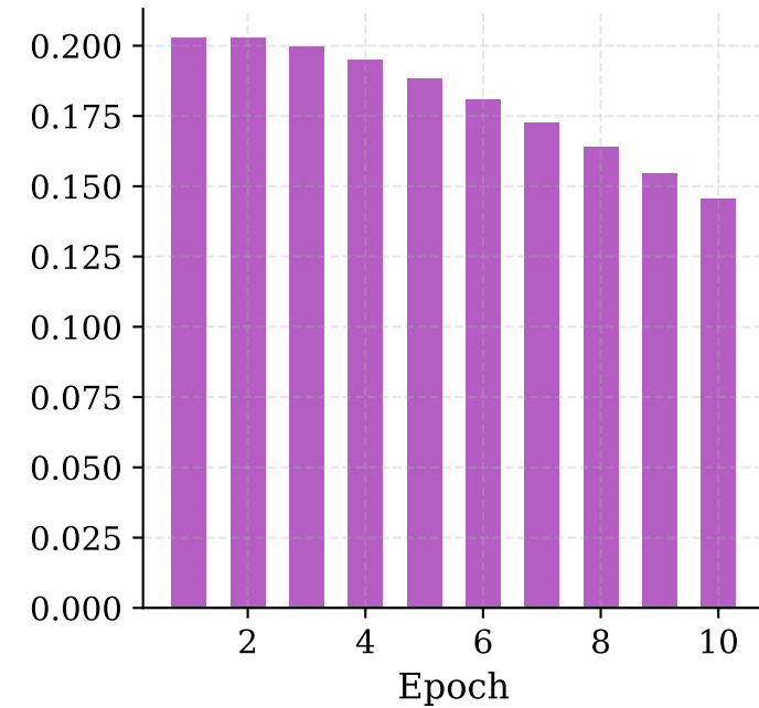
Generalisation Gap
