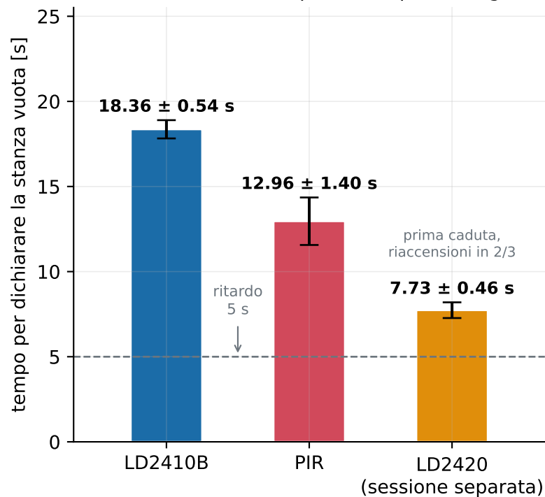
Uscita — 5 trial (3 per l'LD2420) l'LD2410B tiene la presenza più a lungo
