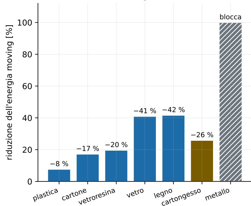
A · LD2410B a 3 m, pannello a 20 cm baseline 53,5 su 6 trial · energia in movimento, scala 0-100
