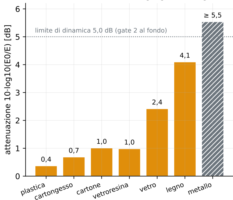
B · LD2420 a 1 m, pannello a 20 cm baseline 39,5 su 6 trial · energia grezza del gate 2
