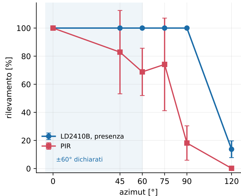
A · LD2410B e PIR, r = 1 m, busto laterale da seduto 3 trial per azimuth, gate max 2
