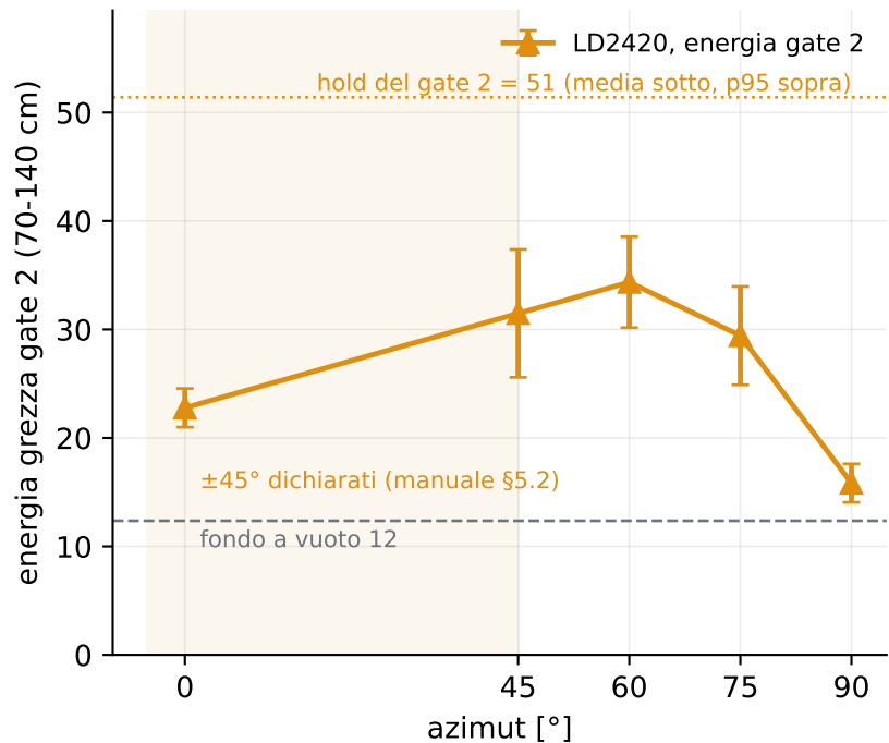
B · LD2420 (esemplare), stessa prova al fondo a 90°: fascio utile fino a \sim 75^\circ
