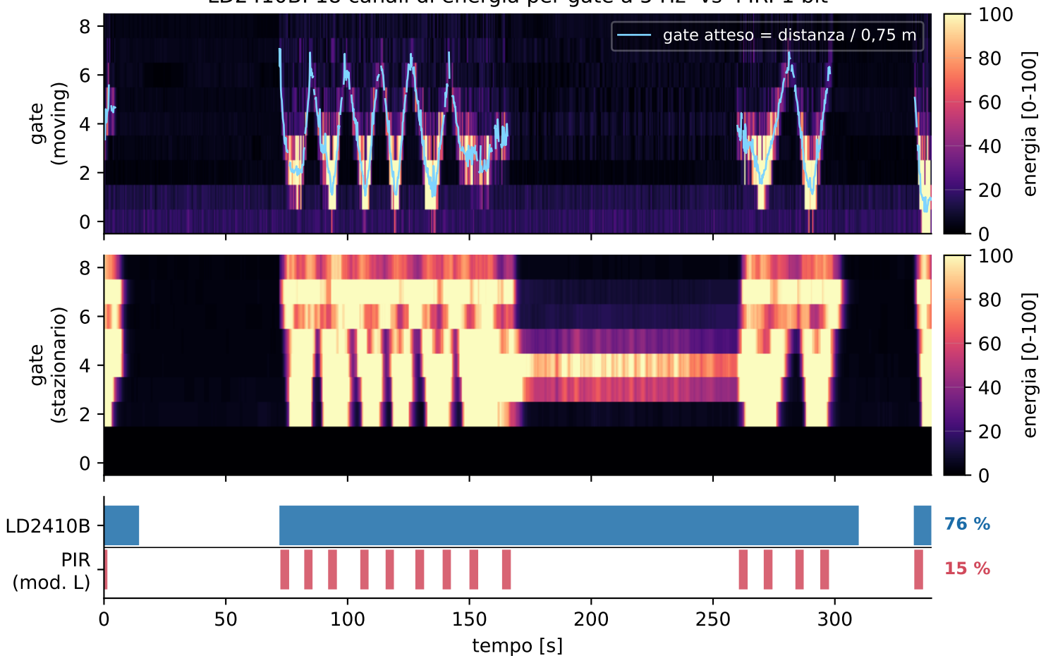
Dati prodotti dai due sensori nello stesso istante LD2410B: 18 canali di energia per gate a 5 Hz vs PIR: 1 bit
