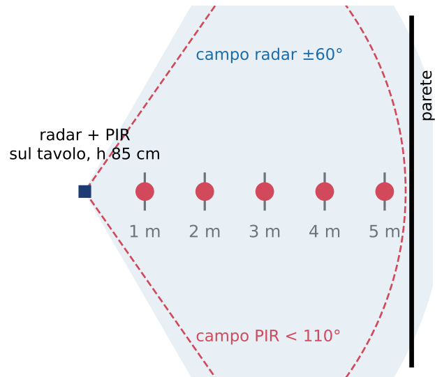
(a) Stanza: tacche a 1-5 m
