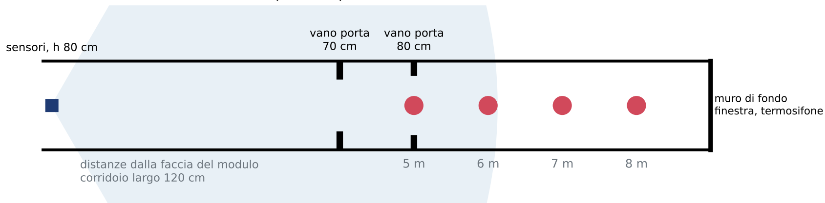
(d) Corridoio della prova di portata: tacche a 5-8 m viste attraverso i due vani
