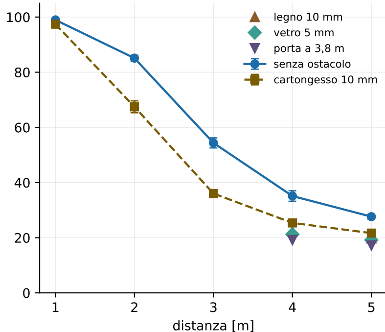
A · LD2410B: energia del bersaglio, pannelli a 20 cm presenza 100 % e distanza corretta in tutti i trial
