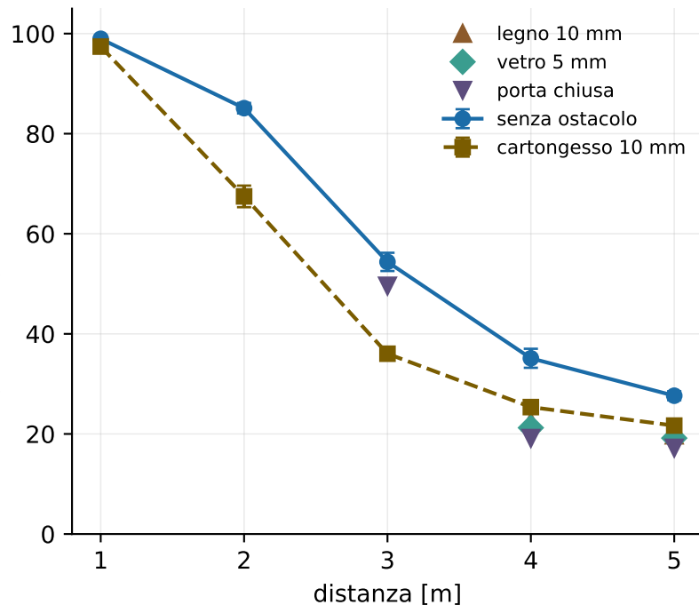
A · LD2410B: energia del bersaglio con l'ostacolo a 20 cm presenza 100 % e distanza corretta in tutti i trial
