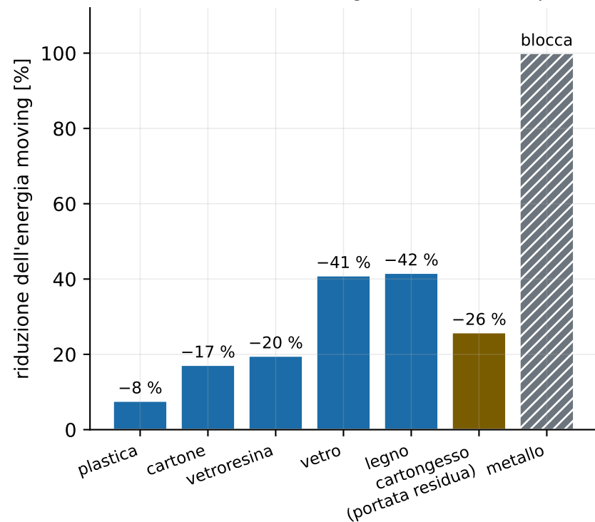
A · LD2410B a 3 m, pannello a 20 cm baseline 53.5 su 6 trial · energia 0-100, non una potenza
