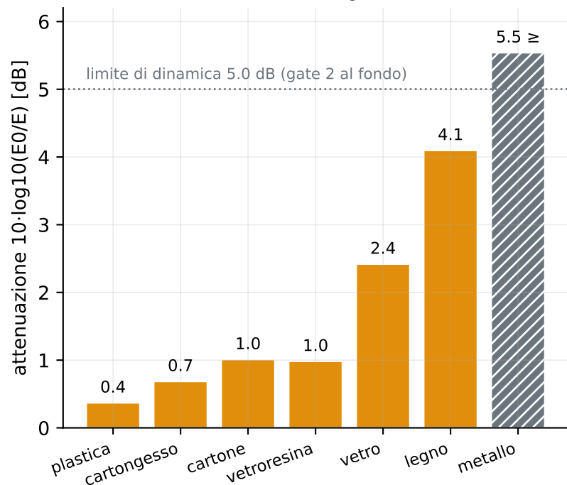
B · LD2420 (esemplare) a 1 m, gate 2 grezzo baseline 39.5 su 6 trial · stessa graduatoria del LD2410B
