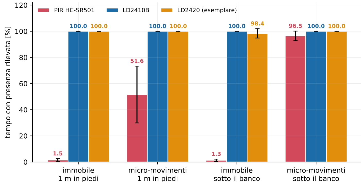
Lo scenario DIPME a tre sensori · 5 trial per condizione stessa geometria per i tre sensori · LD2420 con soglie tarate e scarto iniziale di 90 s
