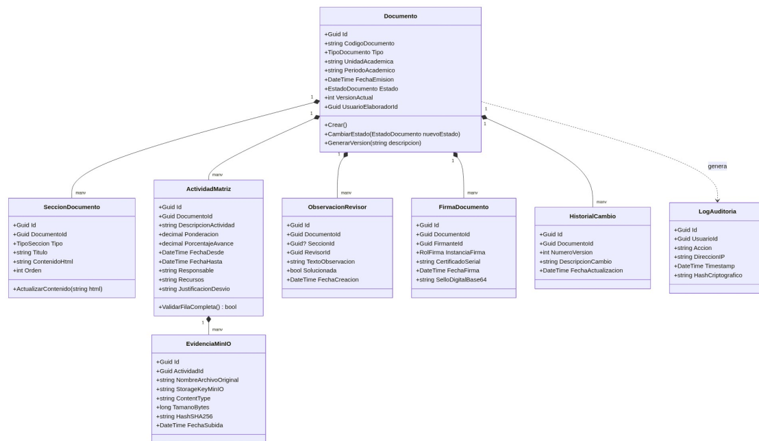
Figura 3: Diagrama de Clases UML del Dominio SIGE.
