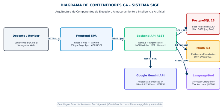
Figura 2: Diagrama de Contenedores del Modelo C4 para el Ecosistema SIGE.
