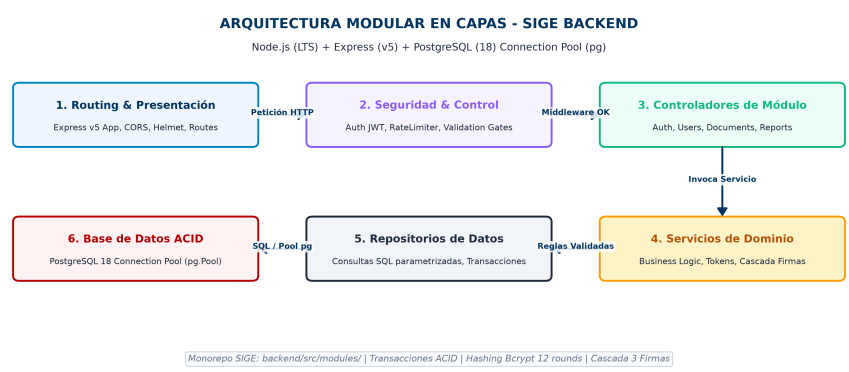
Figura 1: Arquitectura Modular en Capas para Node.js + Express (v5).
