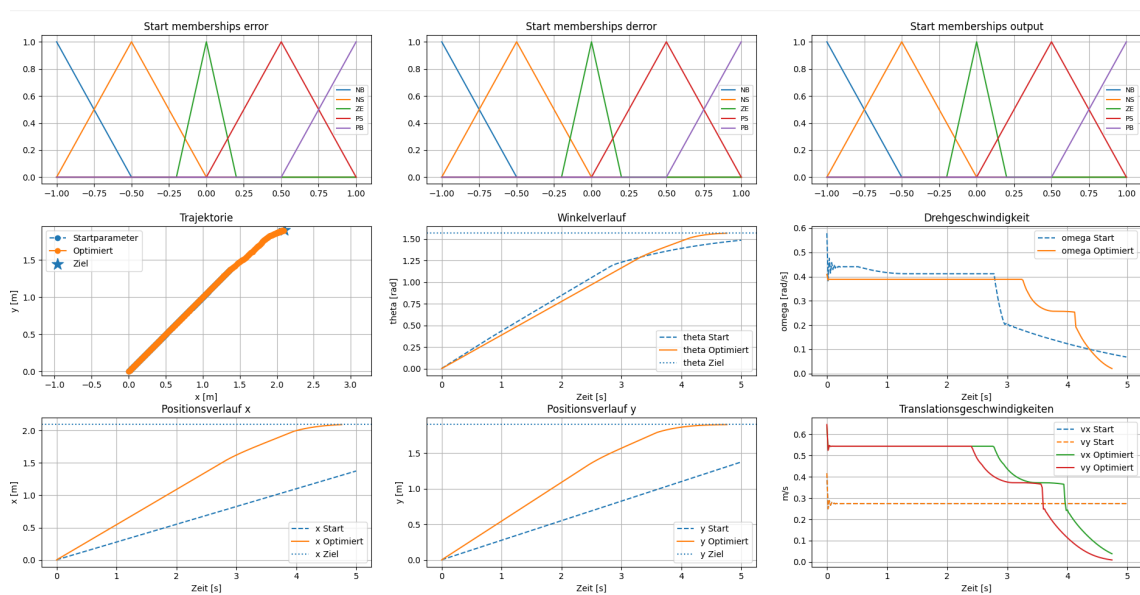
Abbildung 5.2: Gesamtauswertung der Simulation mit Membership-Funktionen, Trajektorie, Winkelverlauf, Positions- und Geschwindigkeitsverläufen.
