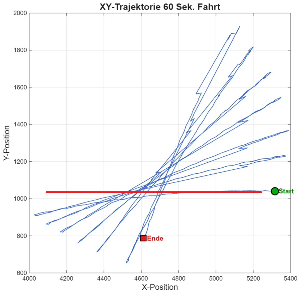
Abbildung 1.1: Ungeregelte Roboterfahrt über 60 Sekunden
