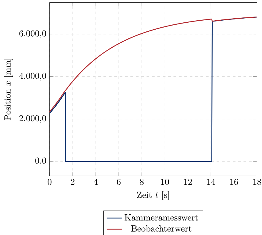
Abbildung 3.9: Gesamtter Zeitverlauf der beobachteten Position mit direktem Ausgleich
