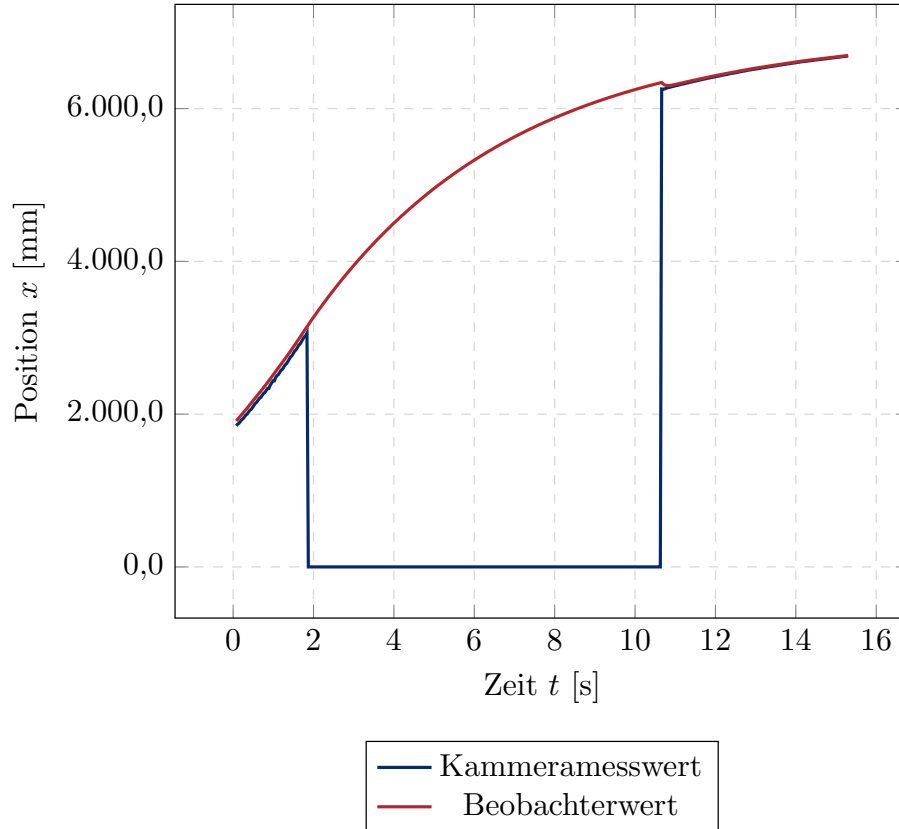
Abbildung 3.12: Beobachter mit variable Verstärkung
