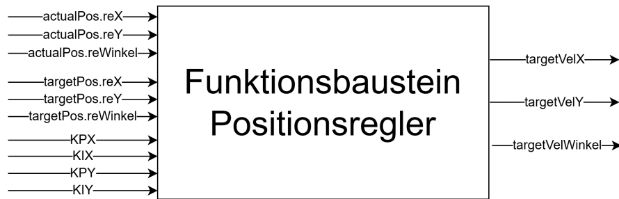
Abbildung 4.3: Positionenregler als Blackbox mit Eingangs- und Ausgangssignalen
