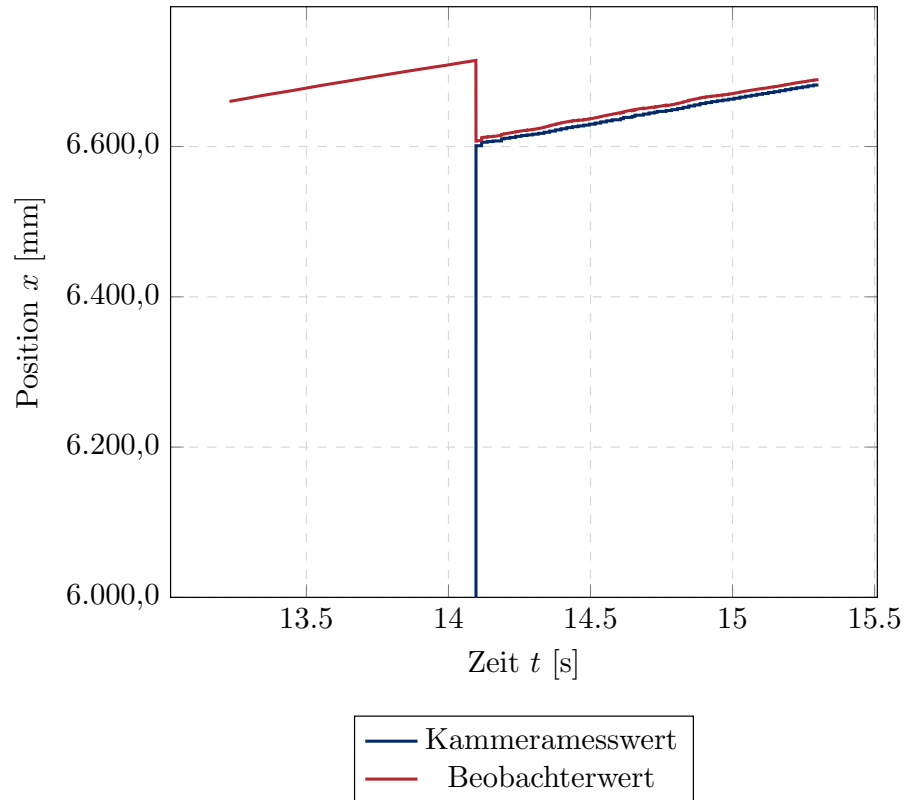
Abbildung 3.10: Ausgleichsvorgang der Position mit direktem Ausgleich
