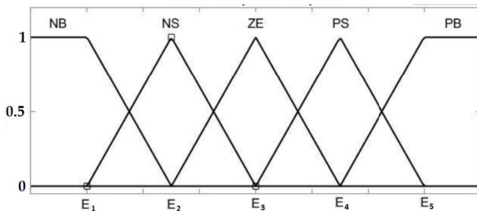
Abbildung 5.1: Schematischer Aufbau von Zugehörigkeitsfunktionen eines Fuzzy-Reglers(übernommen aus [7]).
