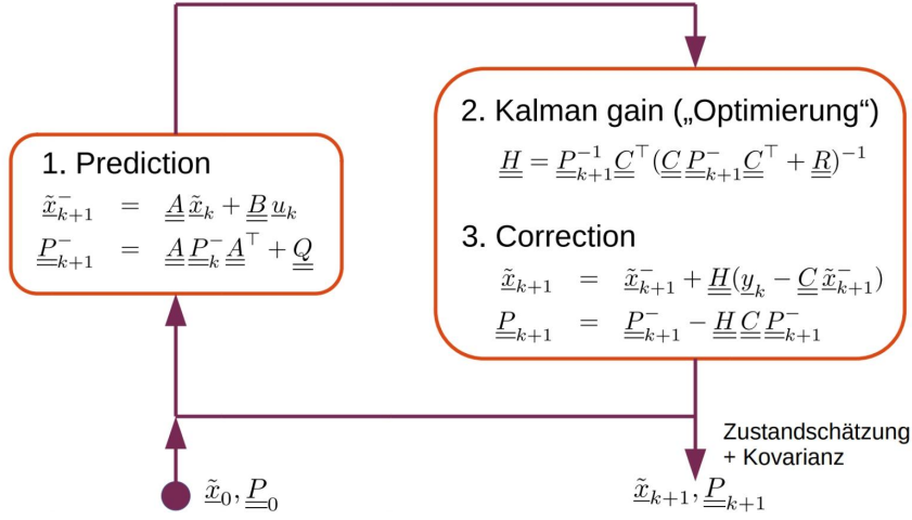
Abbildung 3.6: Konzept Kalman-Filter
