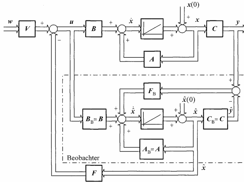
Abbildung 3.5: Zustandsbeobachter nach Luenberger [1]
