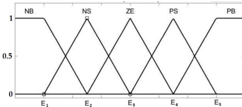
Abbildung 5.1: Schematischer Aufbau von Zugehörigkeitsfunktionen eines Fuzzy-Reglers.
