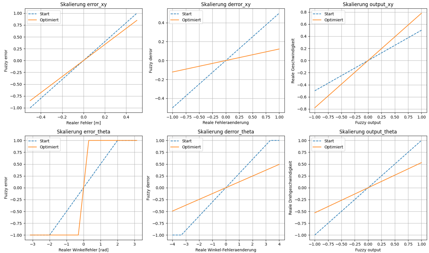
Abbildung 5.3: Vergleich der Start- und Endskalierungen für Positionsfehler, Fehleränderung und Ausgangsgrößen.
