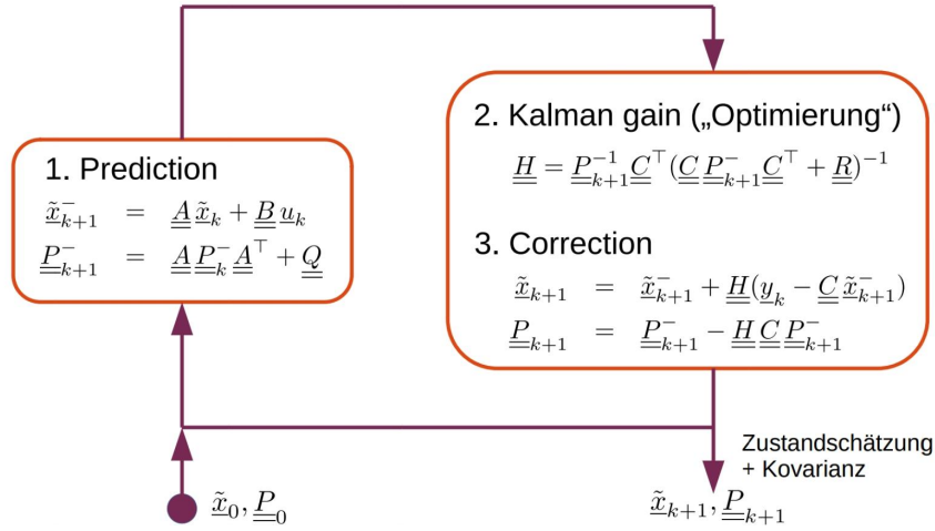
Abbildung 3.6: Konzept Kalman-Filter [1]
