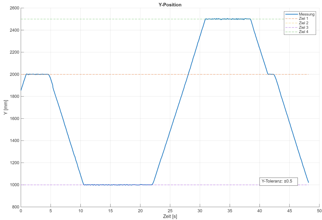
Abbildung 4.15: Rekonstruierte Roboterfahrt in der y-Richtung.
