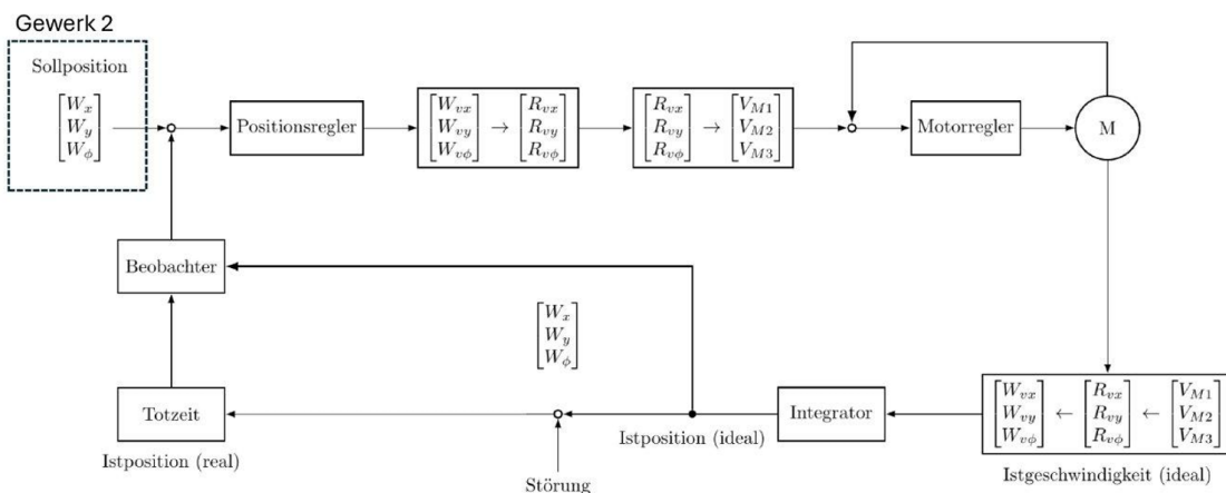
Abbildung 2.2: Blockschaltbild der Positionregelung
