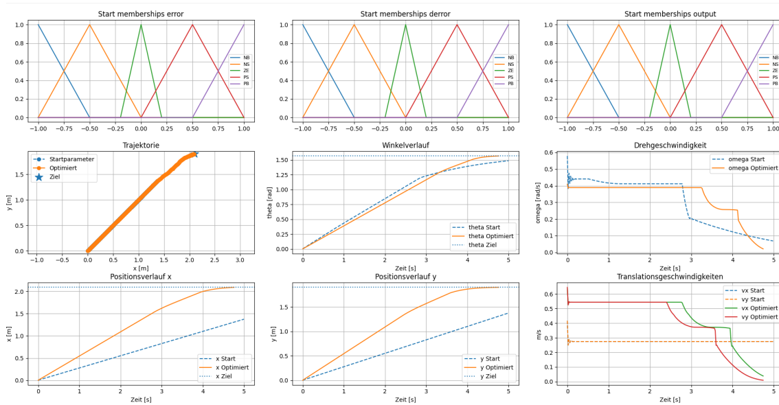
Abbildung 4.12: Gesamtauswertung der Simulation mit Membership-Funktionen, Trajektorie, Winkelverlauf, Positions- und Geschwindigkeitsverläufen.
