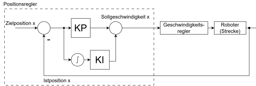
Abbildung 4.4: Interne Struktur des Positionsreglers für die x-Position
