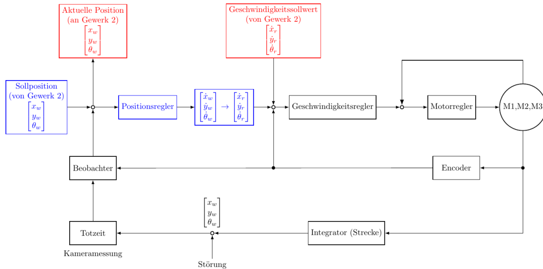
Abbildung 2.1: Blocksaltbild der Bahnregelung. Komponenten der Vektorregelung in rot und Komponenten der Positionsregelung in blau
