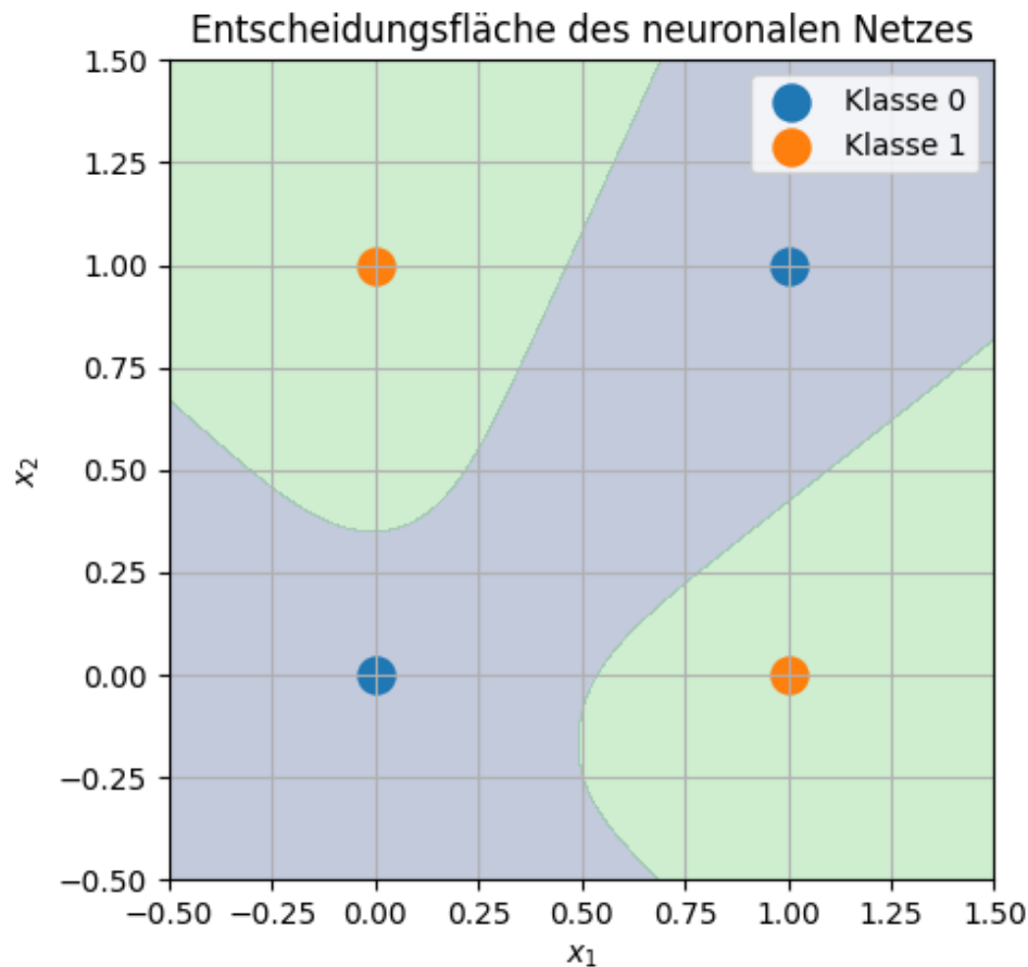
Abbildung 3.10: Entscheidungsfläche des neuronalen Netzes
