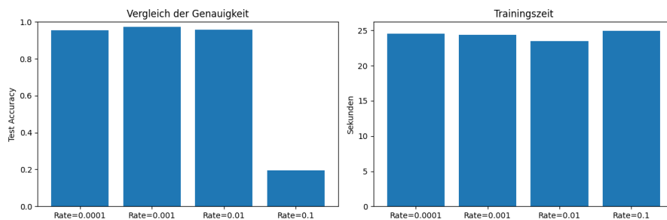
Abbildung 4.6: Vergleich der Genauigkeit und Trainingszeit verschiedener Lernraten.
