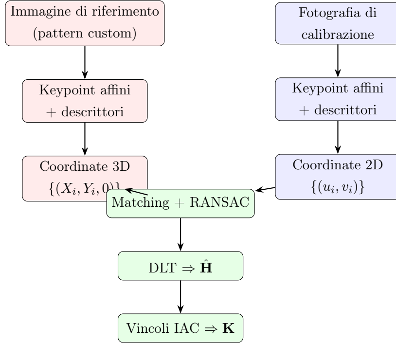
Figura 4: Flusso di costruzione delle corrispondenze con pattern custom. Il ramo rosso (riferimento) e quello blu (fotografia) si fondono nel blocco di matching.
