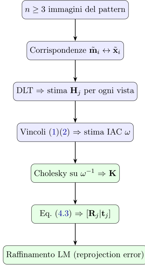
Figura 3: Flusso geometrico del metodo di Zhang. I blocchi verdi producono i parametri finali [5, Fig. 1].
