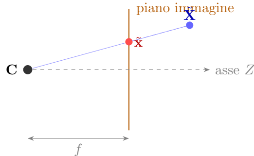
Figura 2: Modello pinhole: \tilde{\mathbf{X}} proiettato su \tilde{\mathbf{x}} attraverso il centro ottico \mathbf{C} a distanza focale f [2, Fig. 6.1].
