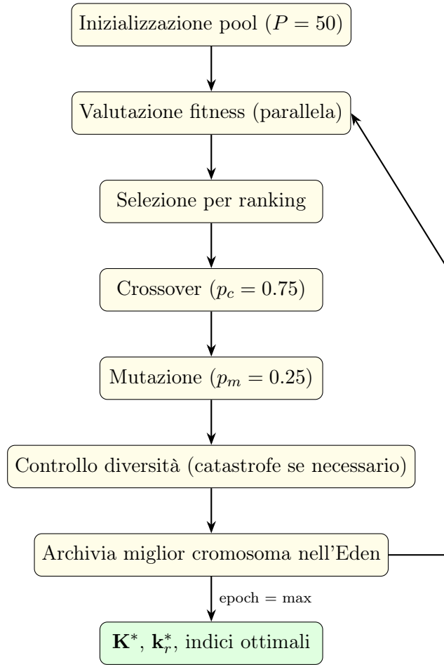
Figura 5: Schema del ciclo evolutivo: il blocco Eden conserva il miglior cromosoma di ogni generazione; al termine si seleziona il miglior Eden.
