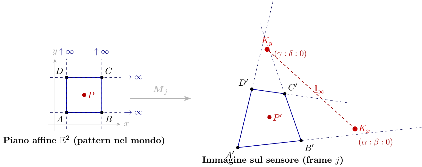
Figura 2: Effetto della proiettività M_j su un quadrato: nel piano affine \mathbb{E}^2 (sinistra) i lati paralleli non si incontrano — corrisponde al pattern planare nel mondo reale. In \mathbb{P}^2 (destra) la proiettività deforma il quadrato in un quadrilatero generico, come appare nell'immagine acquisita; i prolungamenti dei lati convergono ai punti di fuga K_x e K_y , entrambi sulla retta all'infinito l_\infty .
