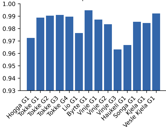
OOF ROC-AUC
