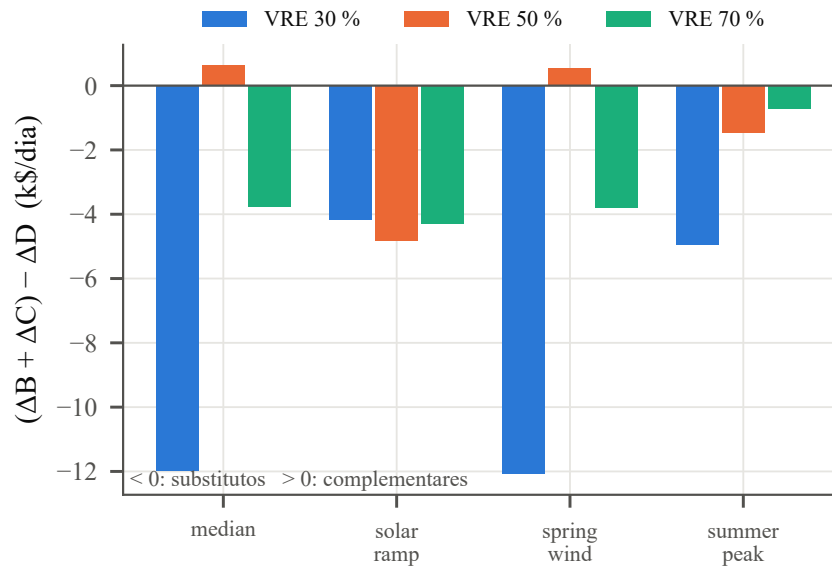
Figura 4: Interação por dia e penetração. Barra negativa indica competição entre os recursos.
