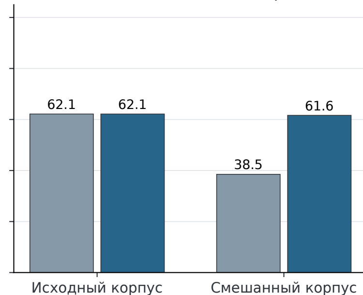
Полнота ссылок · 95 вопросов
