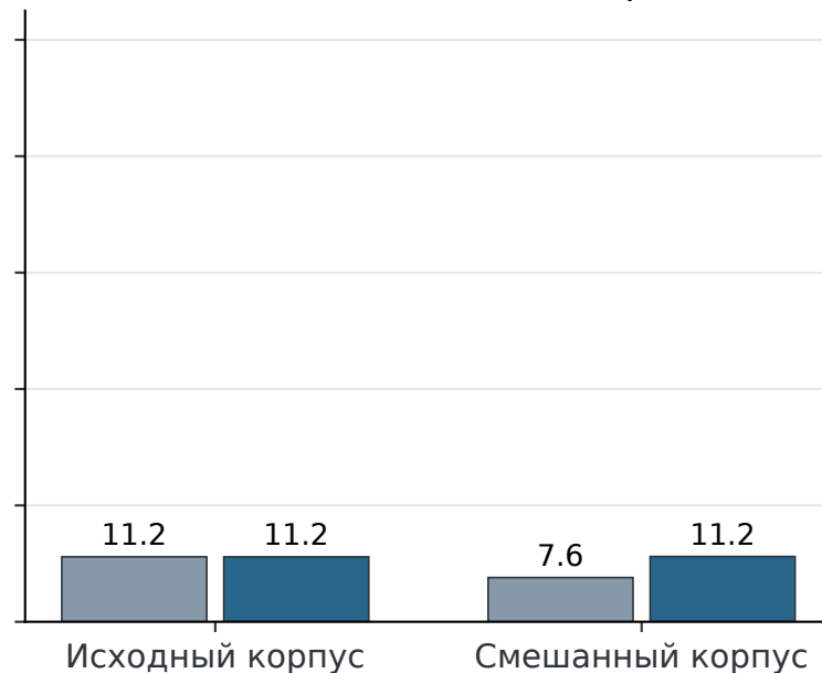
Точность ссылок · 95 вопросов
