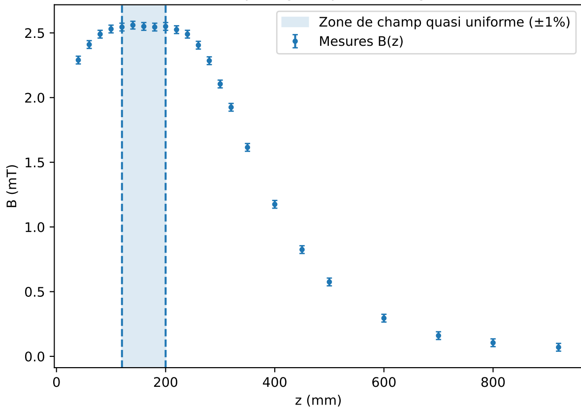
Profil axial du champ magnétique B(z) — grandes bobines
