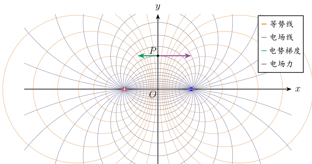
平行带电导线系统电势图
