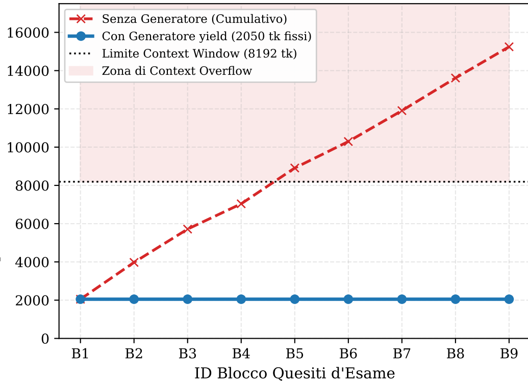
Occupazione Context Window (tk)
