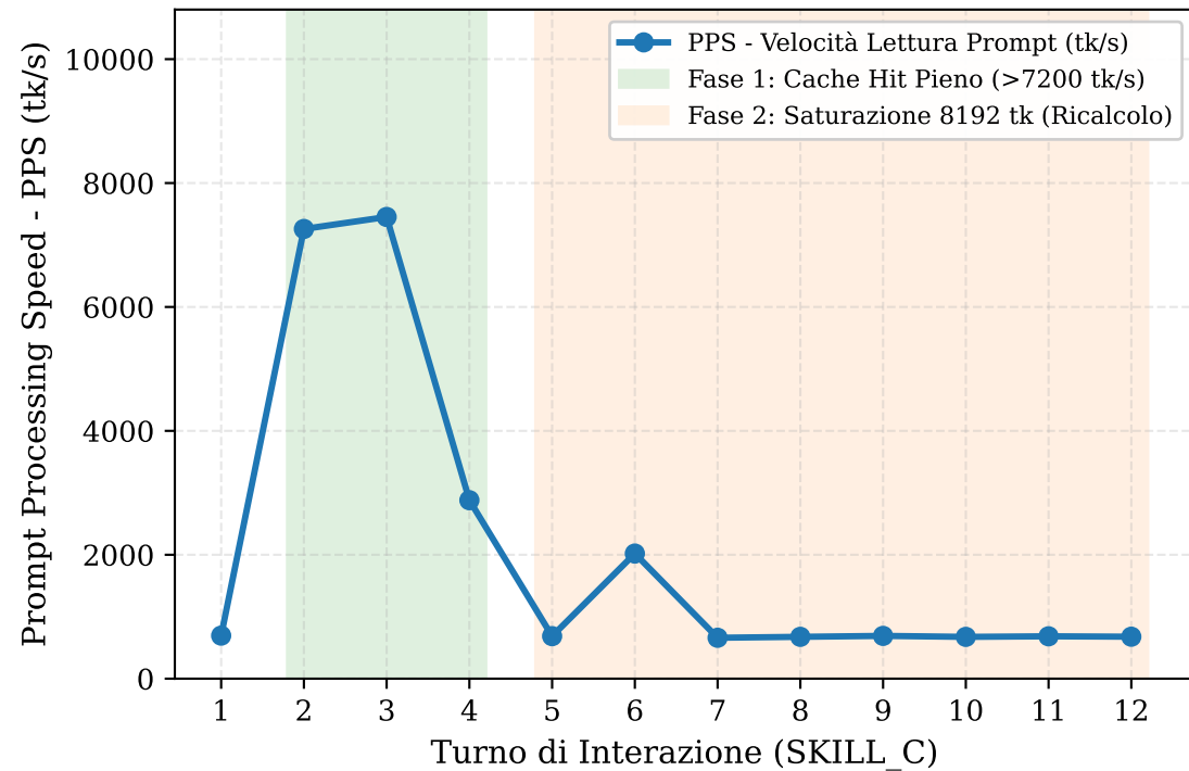
Efficienza del Prefix Caching sulla PPS
