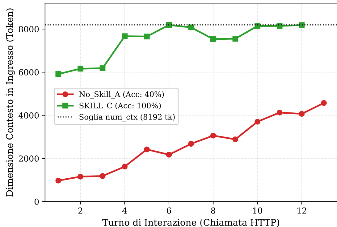
Occupazione della Context Window per Turno
