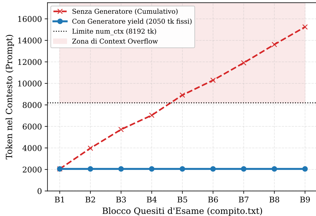
Prevenzione del Context Overflow con yield
