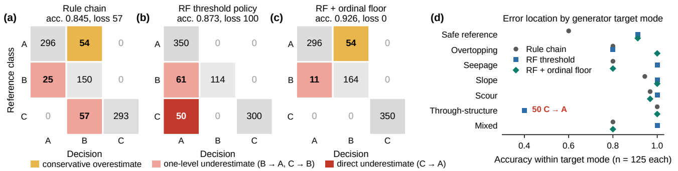
图 2: 875 条受控记录上的错误结构。(a)–(c) 分别为规则链、RF 阈值策略和序数下限混合策略的混淆矩阵; (d) 为各目标模式内的准确率。RF 的所有 C→A 错误均出现在穿结构模式, 该模式所有记录共享一个 14 维特征向量。
