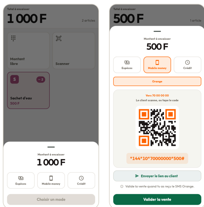
Le choix du mode
