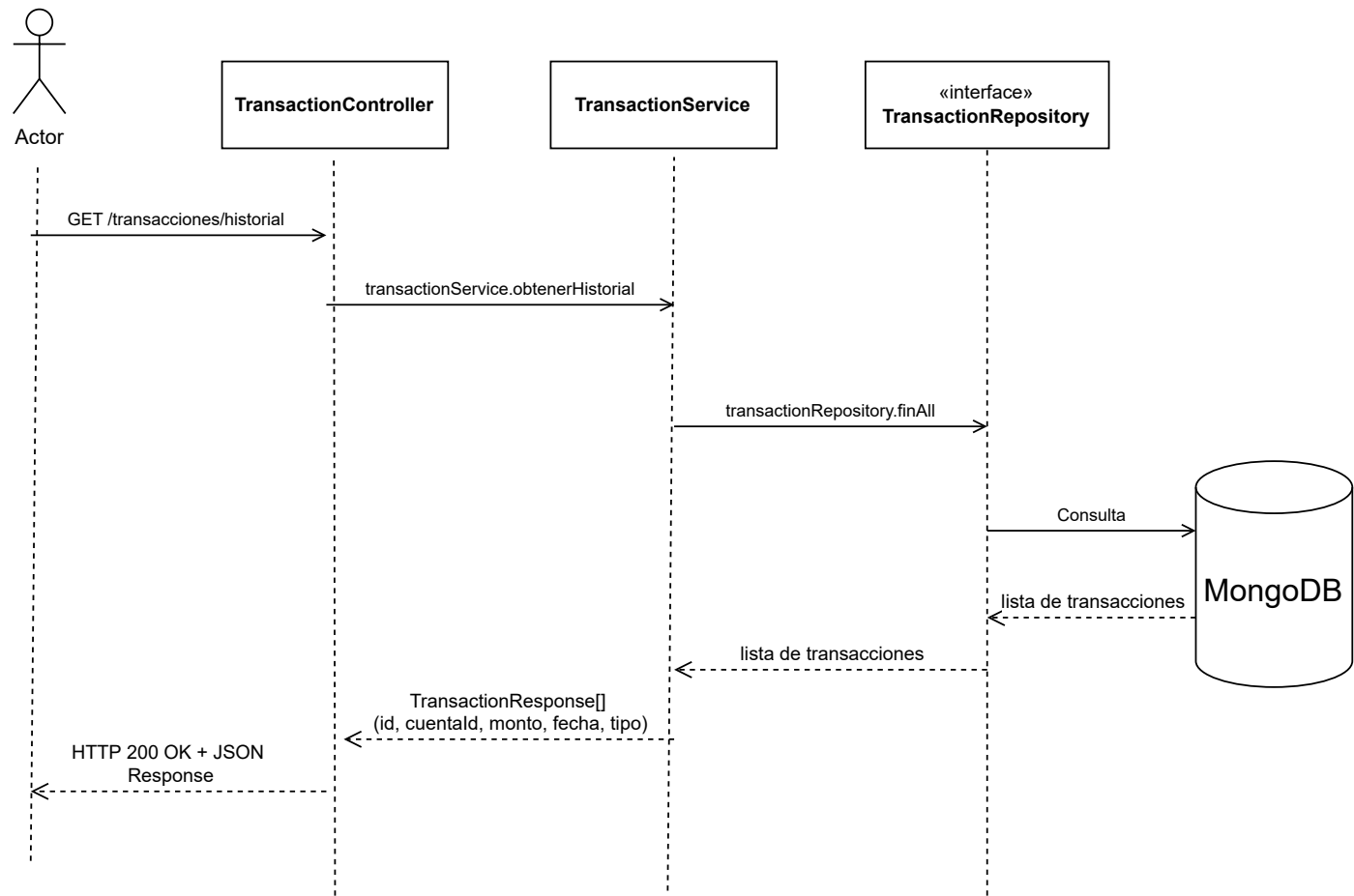
Diagrama de Secuencia GET /transacciones/historial Permite ver el historial
