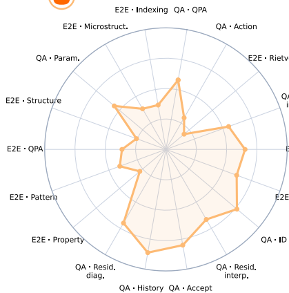
MiMo-V2.5
