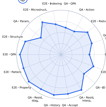
DeepSeek-V4-Flash
