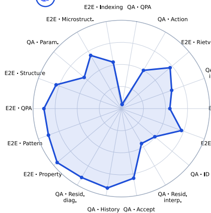
MiniMax-M2.7
