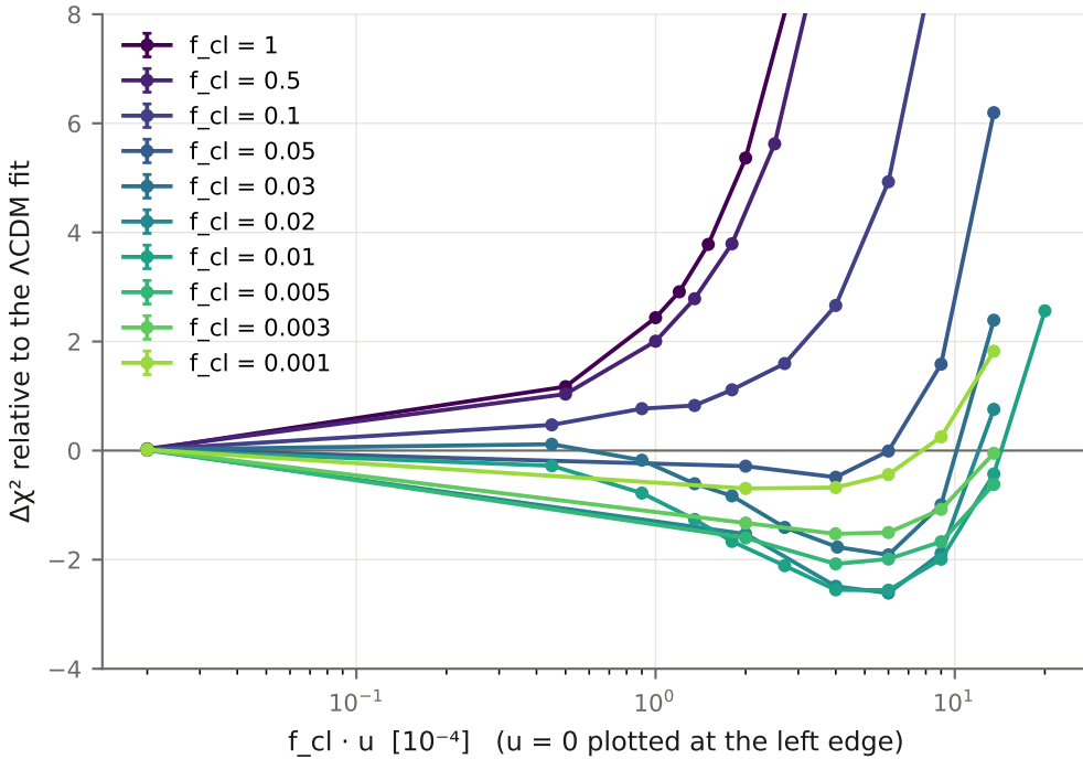
Thomson kernel
