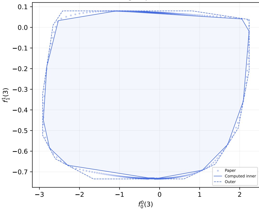
Fig.3: pure S
