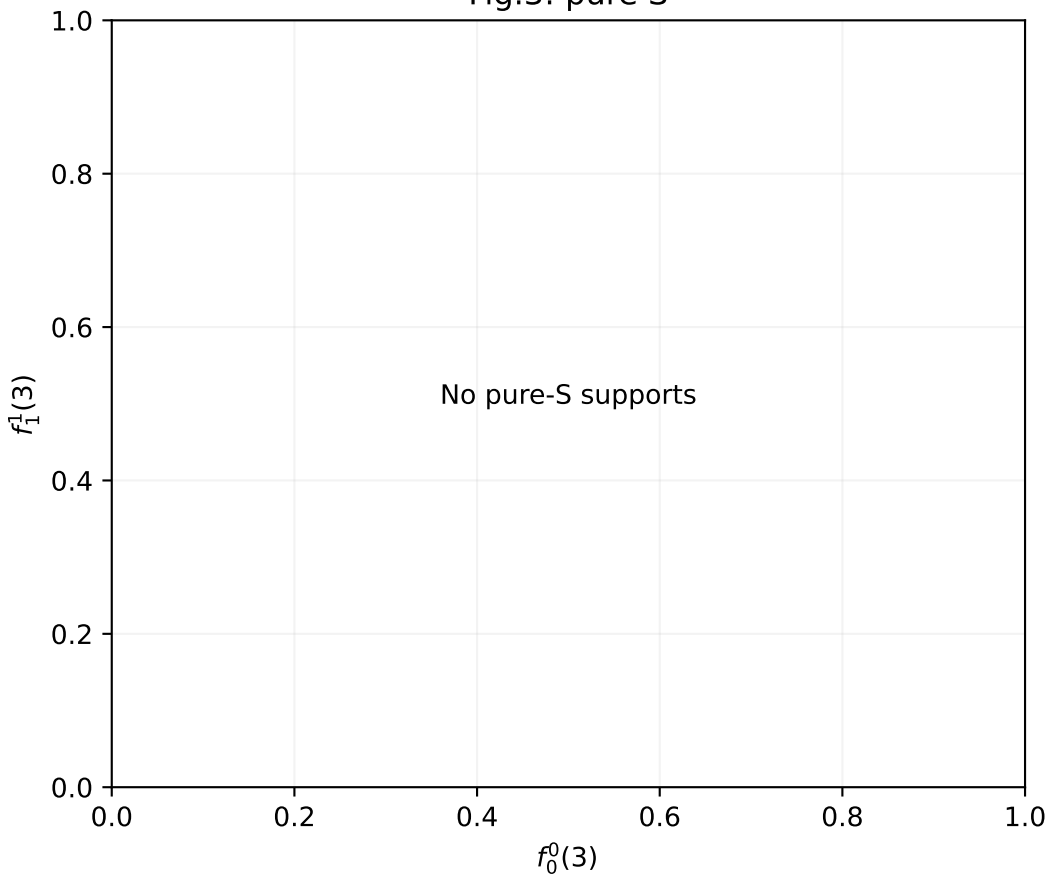
Fig.3: pure S
