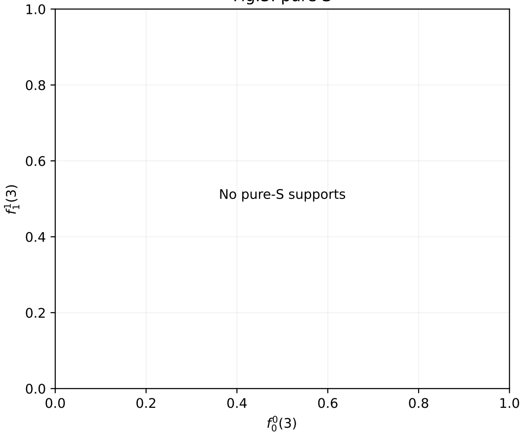
Fig.3: pure S
