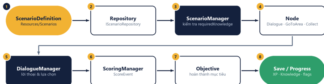
Hình 18.2 — Luồng thực thi kịch bản từ ScenarioDefinition tới lưu tiến trình
