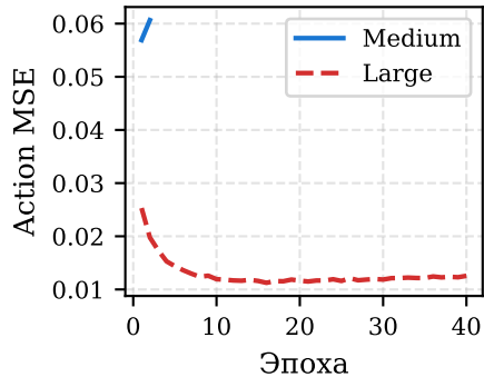
MSE действий \|\hat{a} - a^*\|^2
