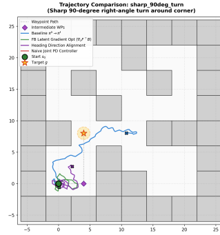
(б) Поворот на 90°: траектории и профиль скорости
