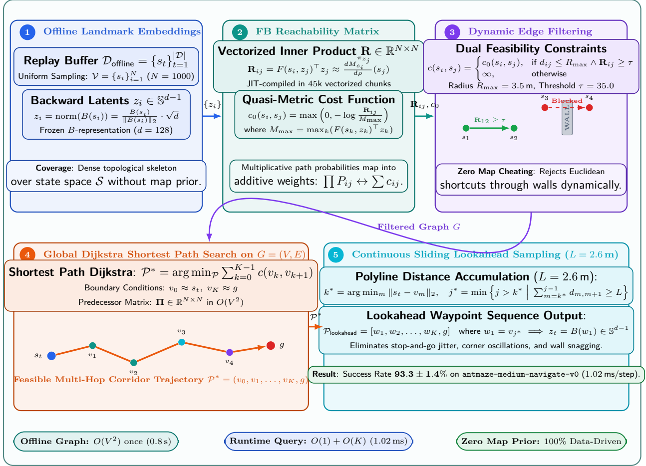
Рис. 2: Построение топологического графа достижимости и алгоритм Дейкстры: (1) Выборка ориентиров из оффлайн-буфера, (2) Фильтрация ребер по FB-достижимости F(s_i, B(s_j))^\top B(s_j) \geq 35.0 без знания карты, (3) Поиск пути Дейкстры и выборка упреждающих вейпоинтов со скользящим окном L = 2.6 м.
