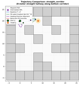
(а) Прямой коридор: траектории и профиль скорости
