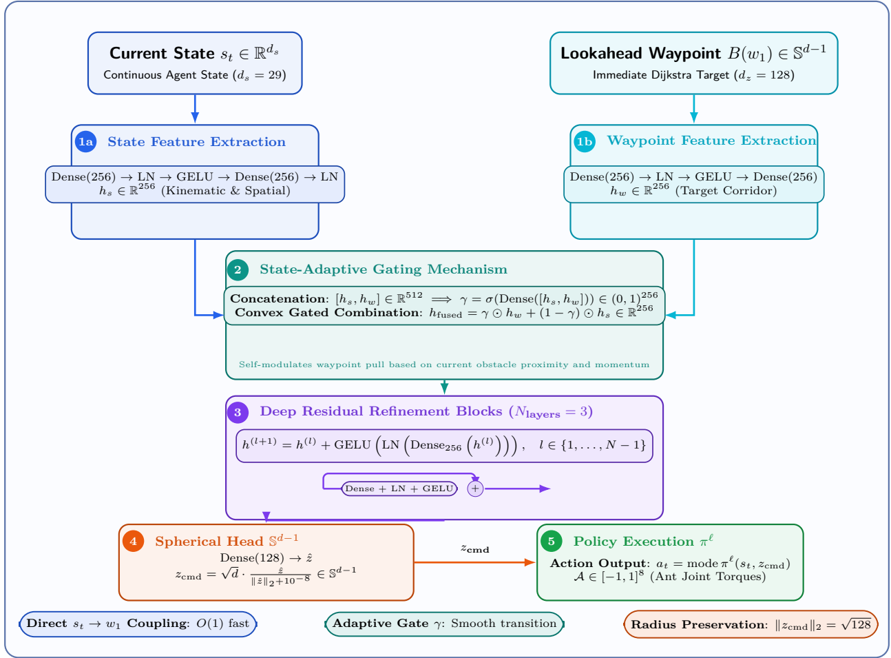
Рис. 4: Архитектура транслятора Single Waypoint Gated Translator: Dual MLP с LayerNorm и GELU, адаптивный гейтинг состояния и ориентира упреждения, глубокие остаточные блоки и выходная проекция z_{\text{cmd}} \in \mathbb{S}^{d-1} напрямую в \pi^\ell .
