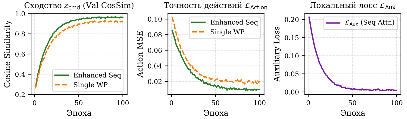
Рис. 8: Сравнение динамики обучения трансляторов: точность предсказания вектора управления z_{cmd} , ошибка действий моторов \mathcal{L}_{Action} и затухание вспомогательного лосса локального якоря \mathcal{L}_{Aux} .
