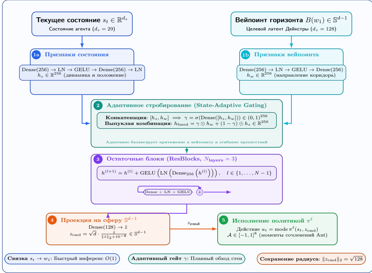
Транслятор одного вейпонта (SingleWaypointTranslator): Gated Residual Архитектура ( s_t, B(w_1) \rightarrow z_{cmd} )
