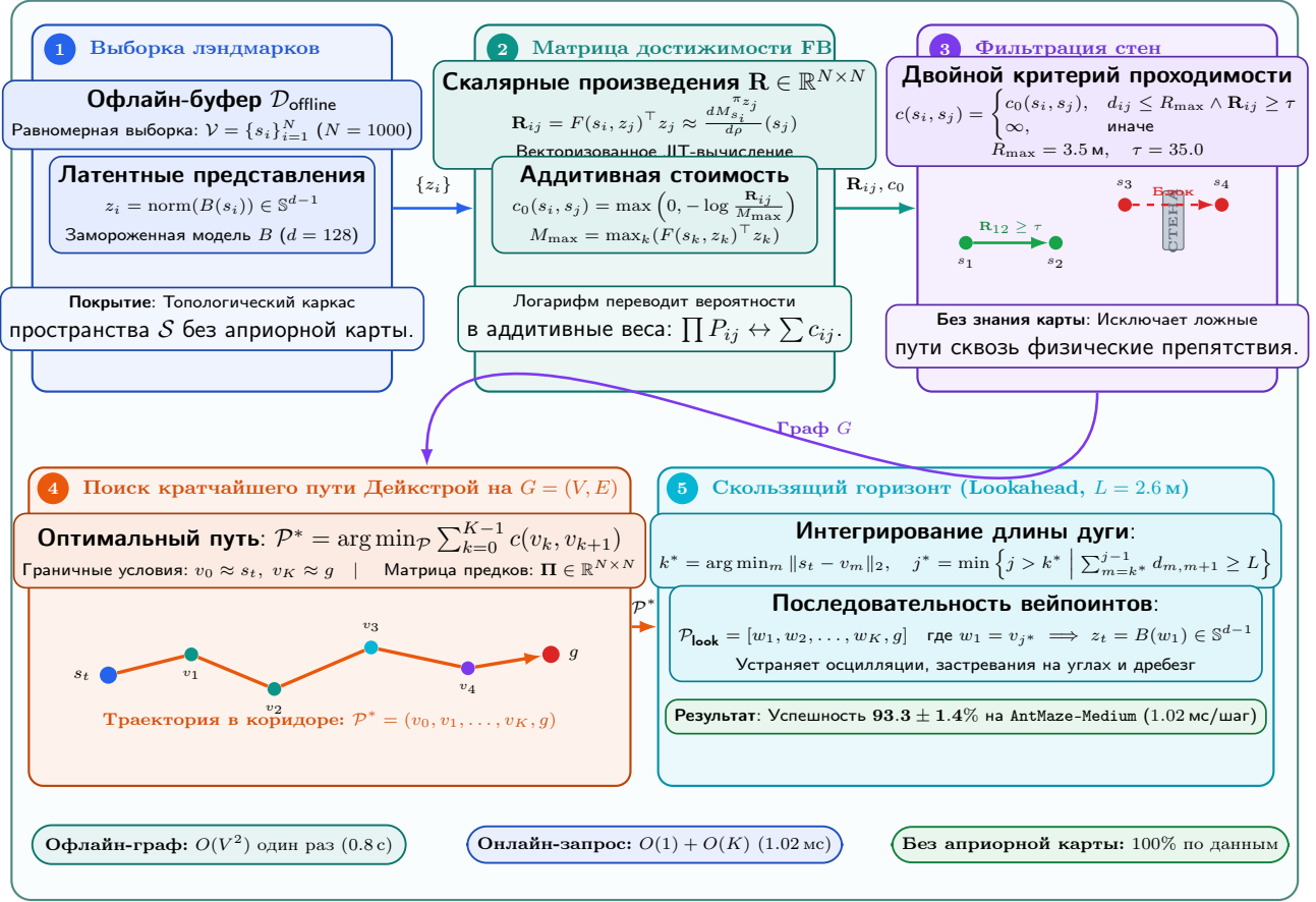
Рис. 2: Построение топологического графа достижимости и алгоритм Дейкстры: (1) Выборка ориентиров из офлайн-буфера, (2) Фильтрация ребер по FB-достижимости F(s_i, B(s_j))^\top B(s_j) \geq 35.0 без знания карты, (3) Поиск пути Дейкстры и выборка упреждающих вейпоинтов со скользящим окном L = 2.6 \text{ м} .
