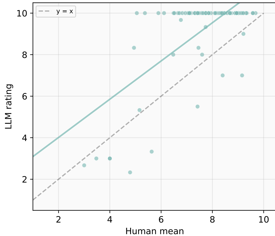
DS-V4-Fl (r=0.66)
