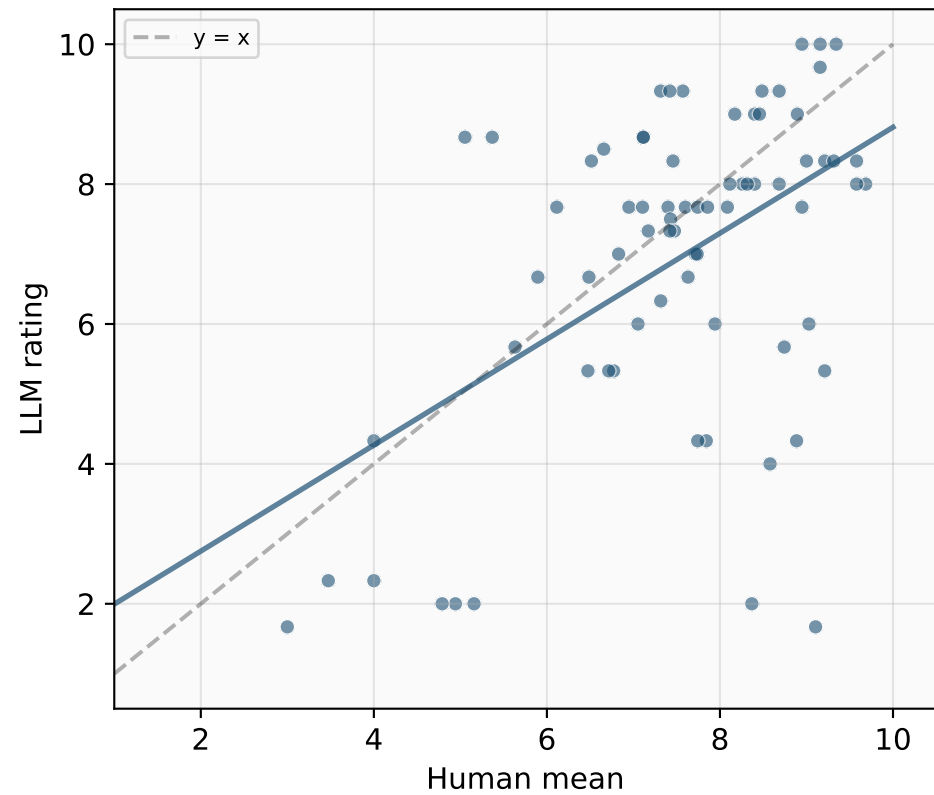
DS-V4-Pro (r=0.51)
