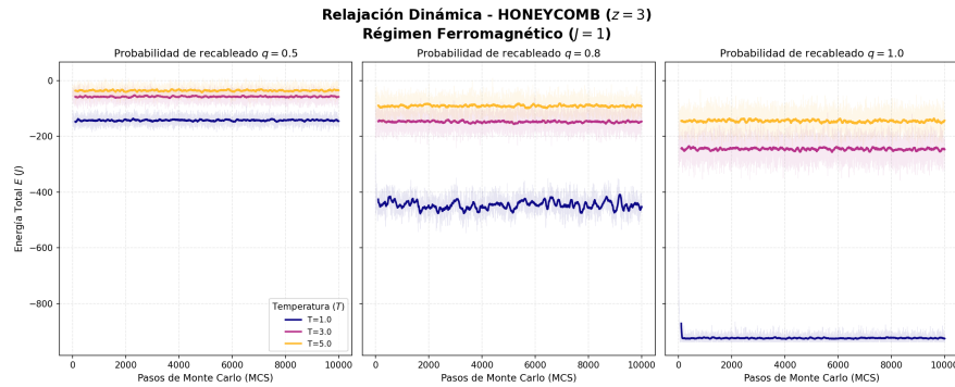
Figura 14: Relajación dinámica de la energía interna E para la red Honeycomb ( z = 3 ) en el régimen ferromagnético ( J = 1 ). Los paneles corresponden a factores de ocupación q = 0.5, 0.8 y 1.0 , con curvas para T = 1.0 (azul), 3.0 (magenta) y 5.0 (amarillo). La escala energética es más amplia que en la cadena 1D. A T = 1.0 se observa una disminución drástica de E al aumentar q , alcanzando su valor mínimo ( \approx -900 ) para q = 1.0 , lo que evidencia una optimización notable del estado de energía en esta geometría al eliminar la dilución.
