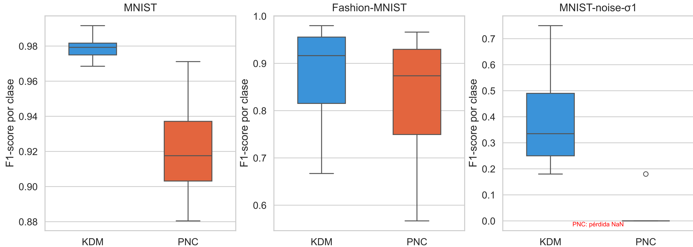
Boxplots de F1-score por Clase: KDM vs PNC
