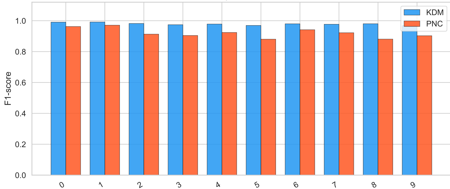
F1-score por Clase: MNIST
