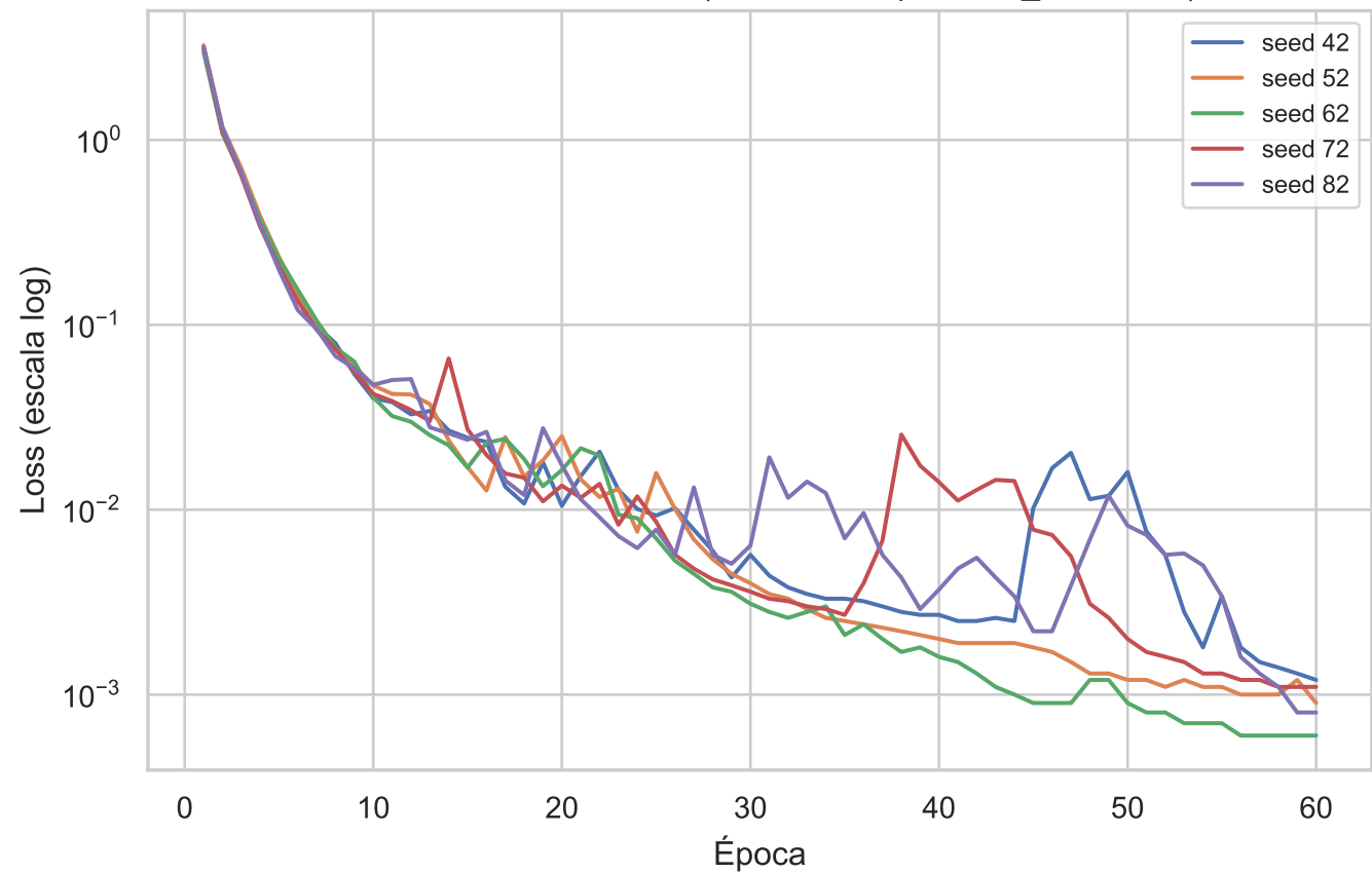
Curvas de entrenamiento (Fase B, 60 épocas, lr_kdm=3e-3)
